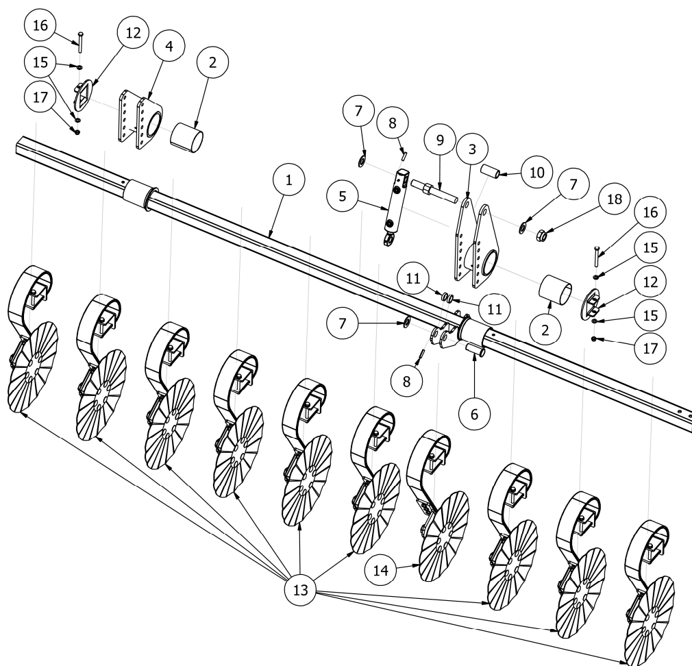
Rysunek R6 BT01559 Belka talerzy tnących prawa BM
