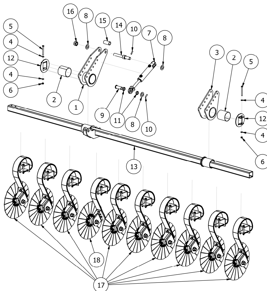
Rysunek R7 BT01538 Belka talerzy tnących lewa BM
